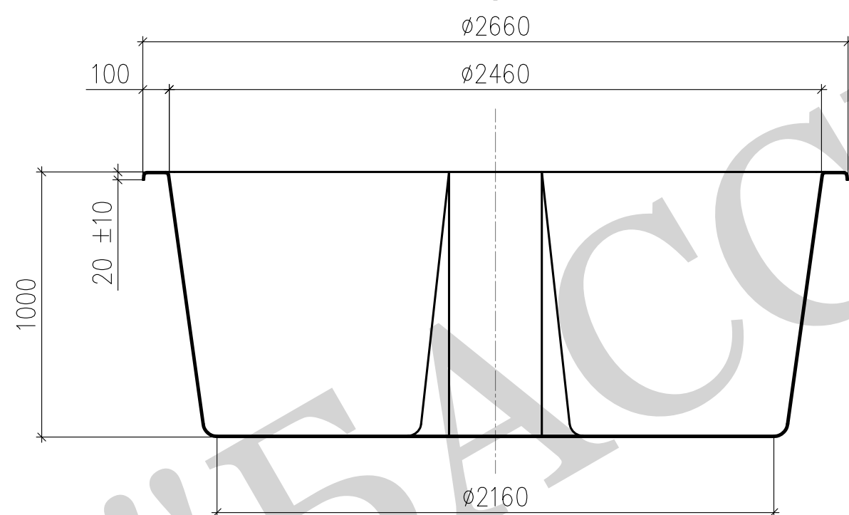
Вид А
