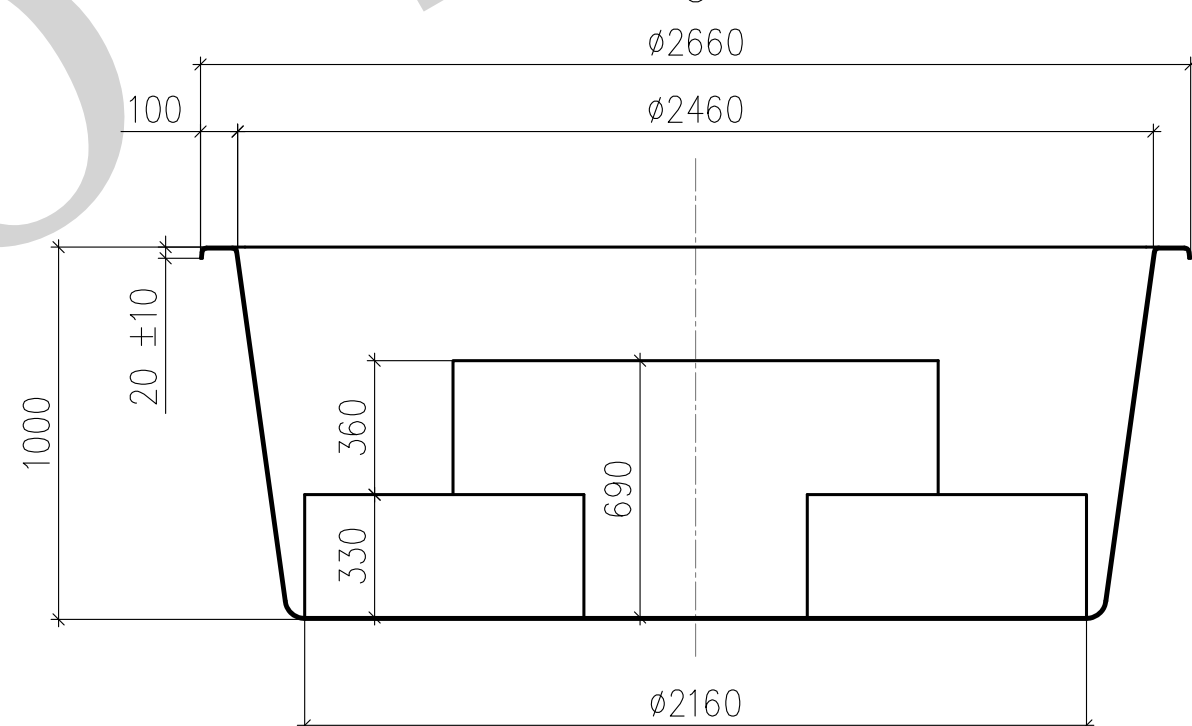
Вид Б
